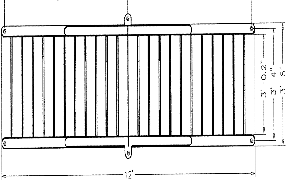
V2 TOP VIEW P-1
